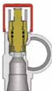
Рис. 20. Запорно-балансировочный коллектор
